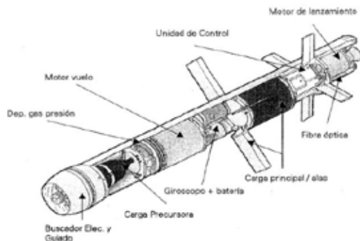
Foto: Estructura del misil Spike LR. Fuente: Ministerio de Defensa 263
